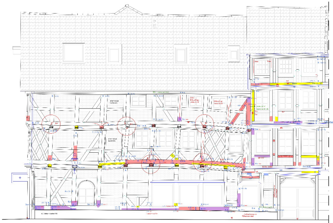
Bild 4: Auszug aus Schadenskartierung in verformungstreuer Bauaufnahme 2023: Trauffassade Fachwerkgebäude Am Markt 5
